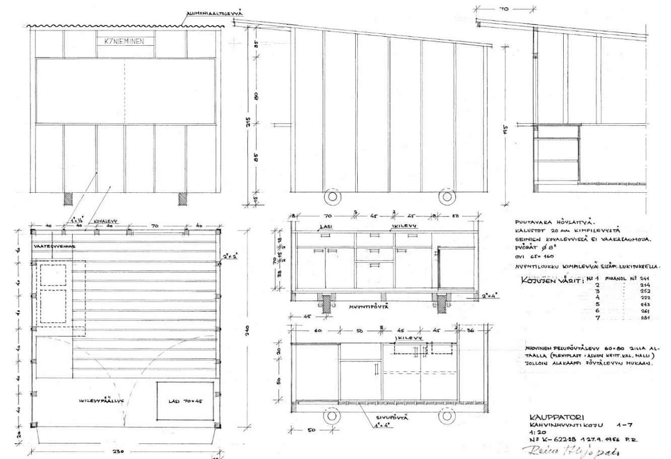
Kuva 32. Vuonna 1956 suunnitellut kahvimyyntikojut (Reino Ahjopalo). Lähde: LKA
