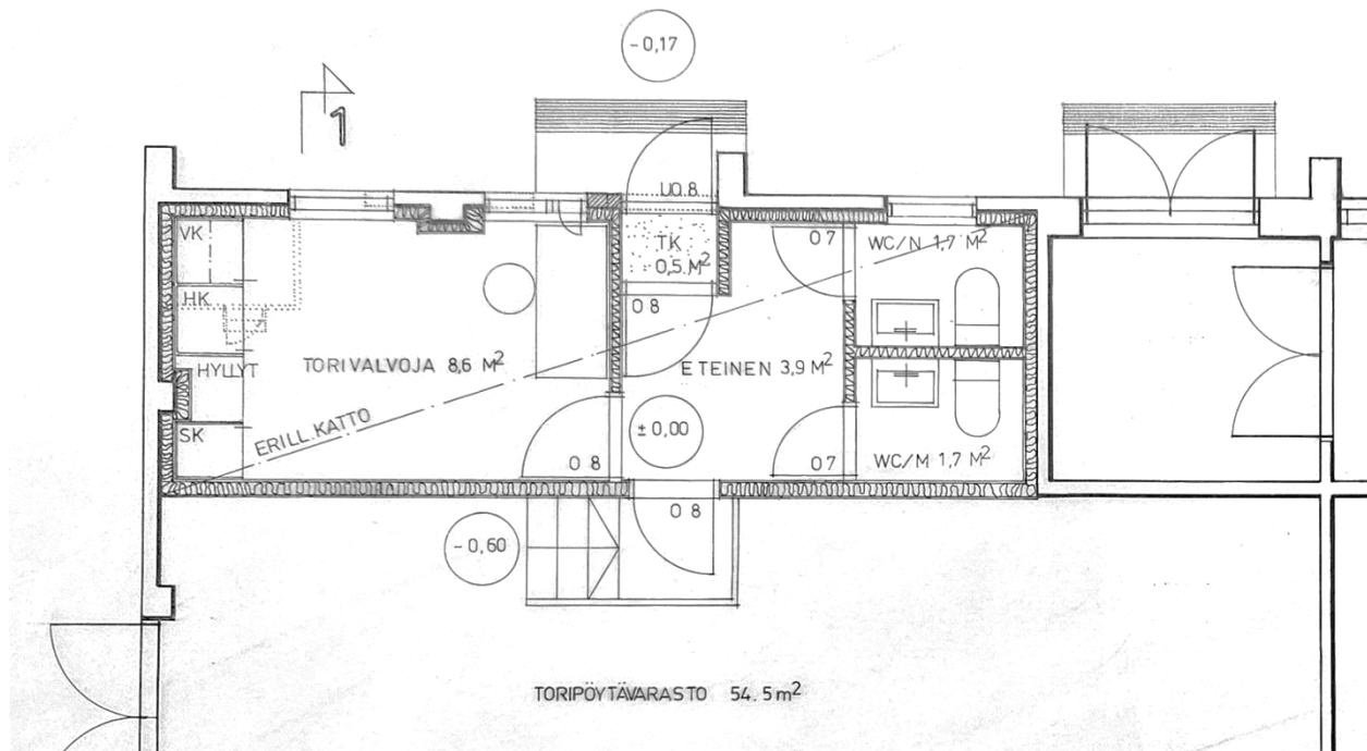
Kuva 54. Vuonna 1977 toripöytävaraston tiloihin suunniteltu torivalvojan ja -myyjien sosiaalitilat. Julkisivuun on lisätty uusi ulko-ovi ja kaksi ikkunaa uusittu. Torivalvojan koppi on poistettu. Lähde: LKA
