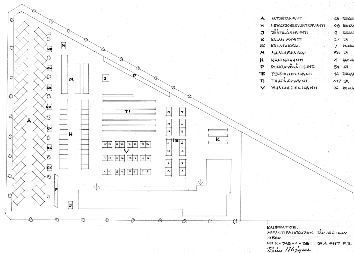
Kuva 31. Alkuperäinen kauppatorin myyntipaikkojen järjestely vuodelta 1957. Seitsemän kahvinmyyntikojua oli tällöin paikoillaan. Piirustuksen on signeerannut kaupunginarkkitehti Reino Ahjopalo. Lähde: LKA
