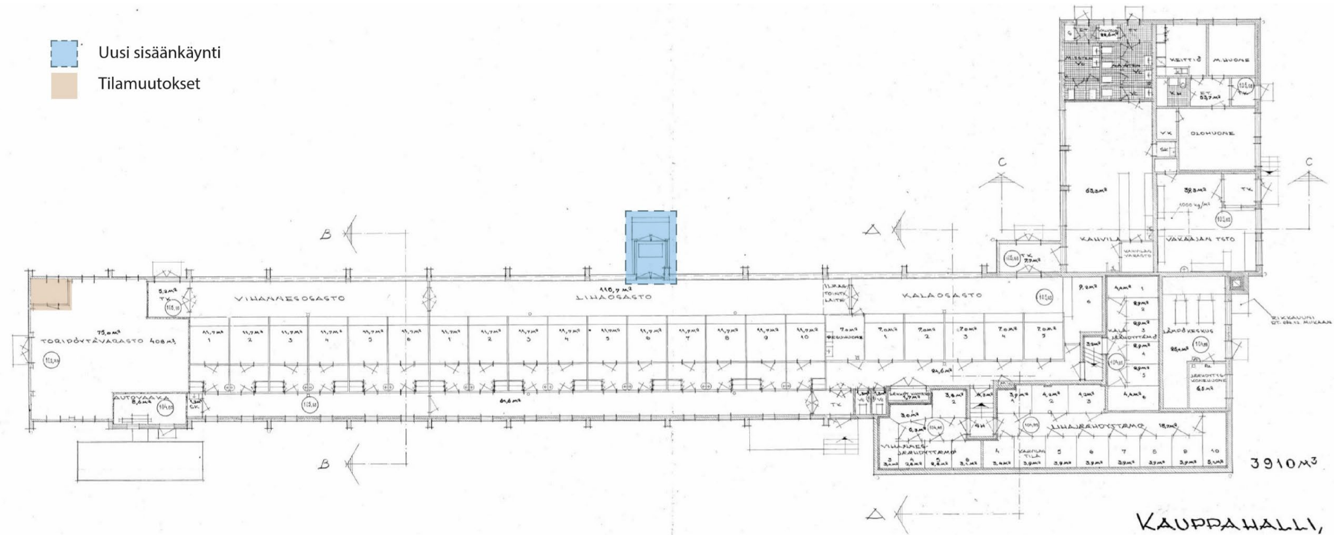
Kuva 52. Muutoksia vuonna 1967. Alkuperäiseen suunnitelmaan lisätty uusi sisäänkäynti torin puolelle ja toripöytävarastoon rakennettu torivalvojan koppi. Lähde: LKA
