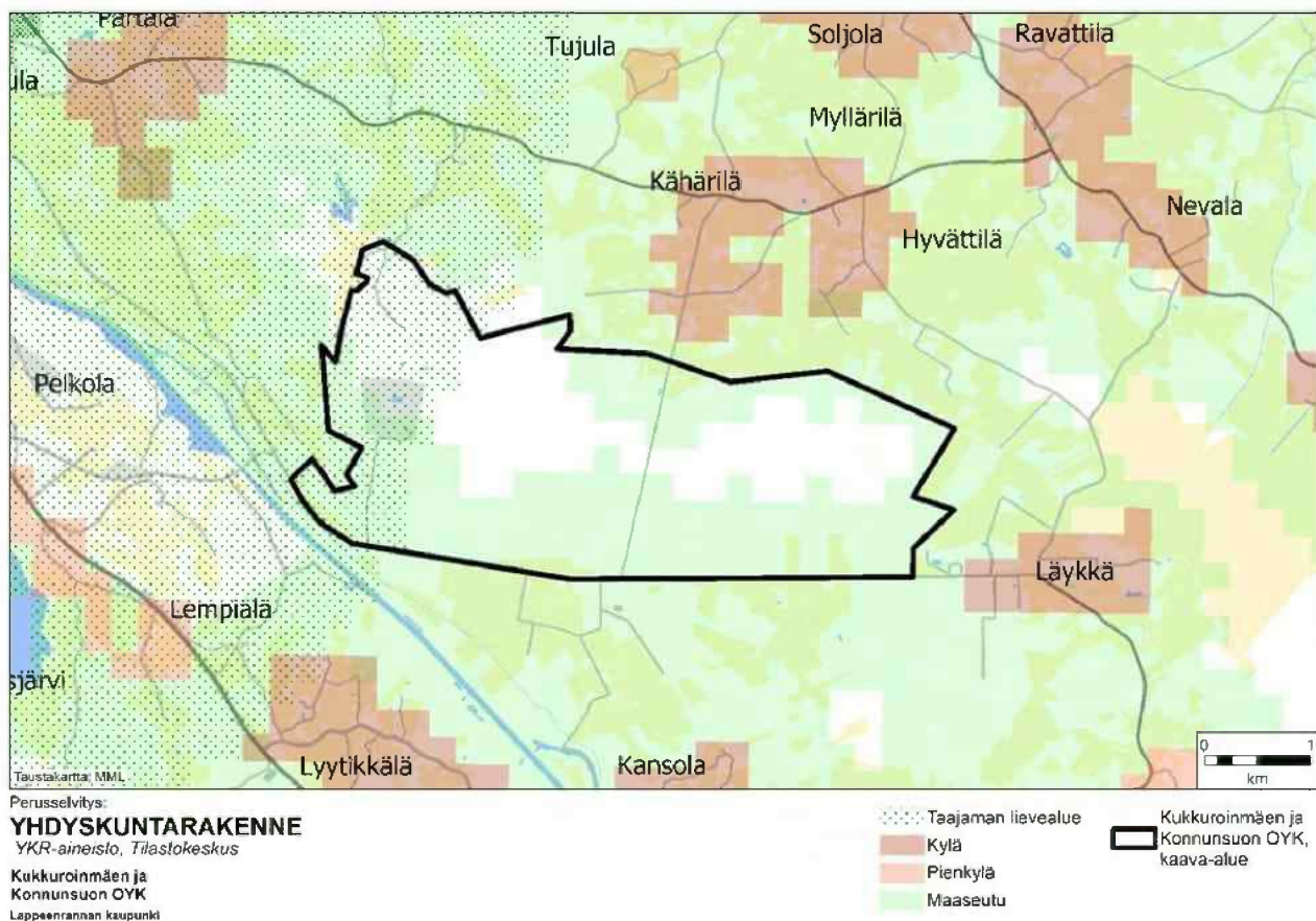
Kuva 7. Yhdyskuntarakenne (Tilastokeskus 2017).
