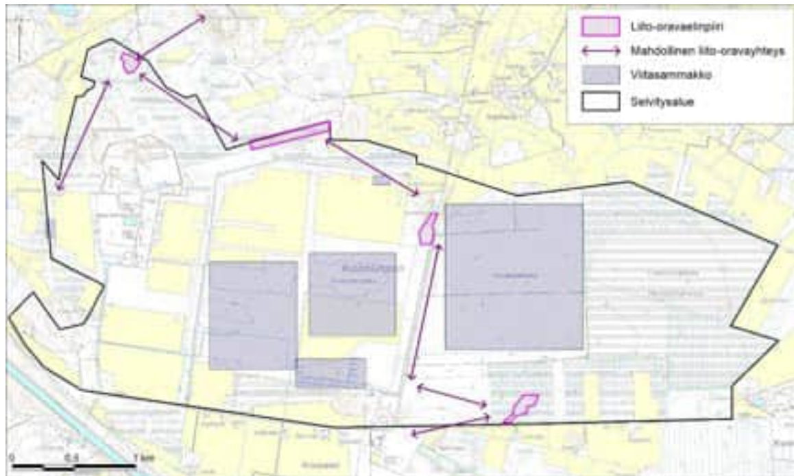
Kuva 14. Luontodirektiivin liitteen IV (a) lajien liito-oravan elinyriit ja viitasammakoiden kutupaikka-alueet vuonna 2022. Hyvättilänsuon luonnonsuojelualuetta itäosassa ei kartoitettu.
