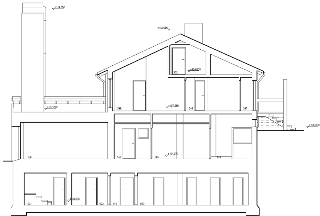
LEIKKAUS A - A
