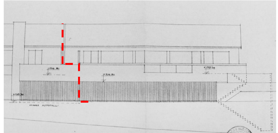
Kuva: Vuonna 1966 valmistuneen laajennusosan länsifasadi. Yläkerrassa on parveke ja II kauppalanlääkärin asunto, alakerrassa väestönsuojakeskus. Vanhan (vasemmalla) ja uuden puolen raja merkitty kuvaan katkoviivalla. / Rakennuspiirustus 28.9.1965. LKA
