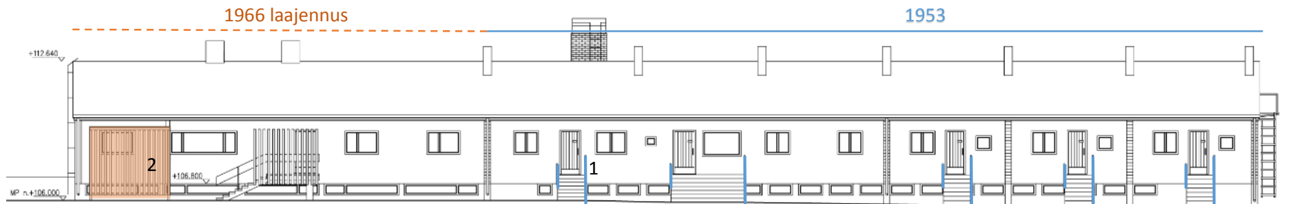
Fasadi itään, 28.8.1952. Martikainen & Ypyä. LKA.
