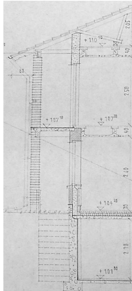
Kuva: Vuonna 1953 valmistuneen terveystalon leikkauskuva: tiili-, kevyttiili- ja betonirakenteet, huonekorkeudet ja kattotuolit. / Martikainen / Ypyä 28.8.1952. LKA
